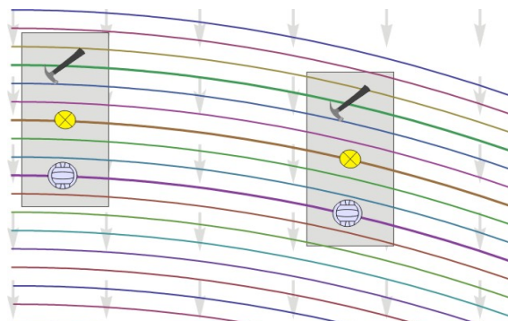
Abb. 1: Schwerelosigkeit im homogenen Gravitationsfeld: Die Wurfparabeln von Ball und Hammer verlaufen parallel zu der des Kasten-Schwerpunkts.
